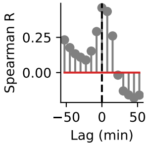
Uracil
