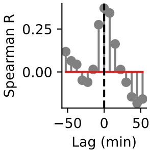
Xanthine
