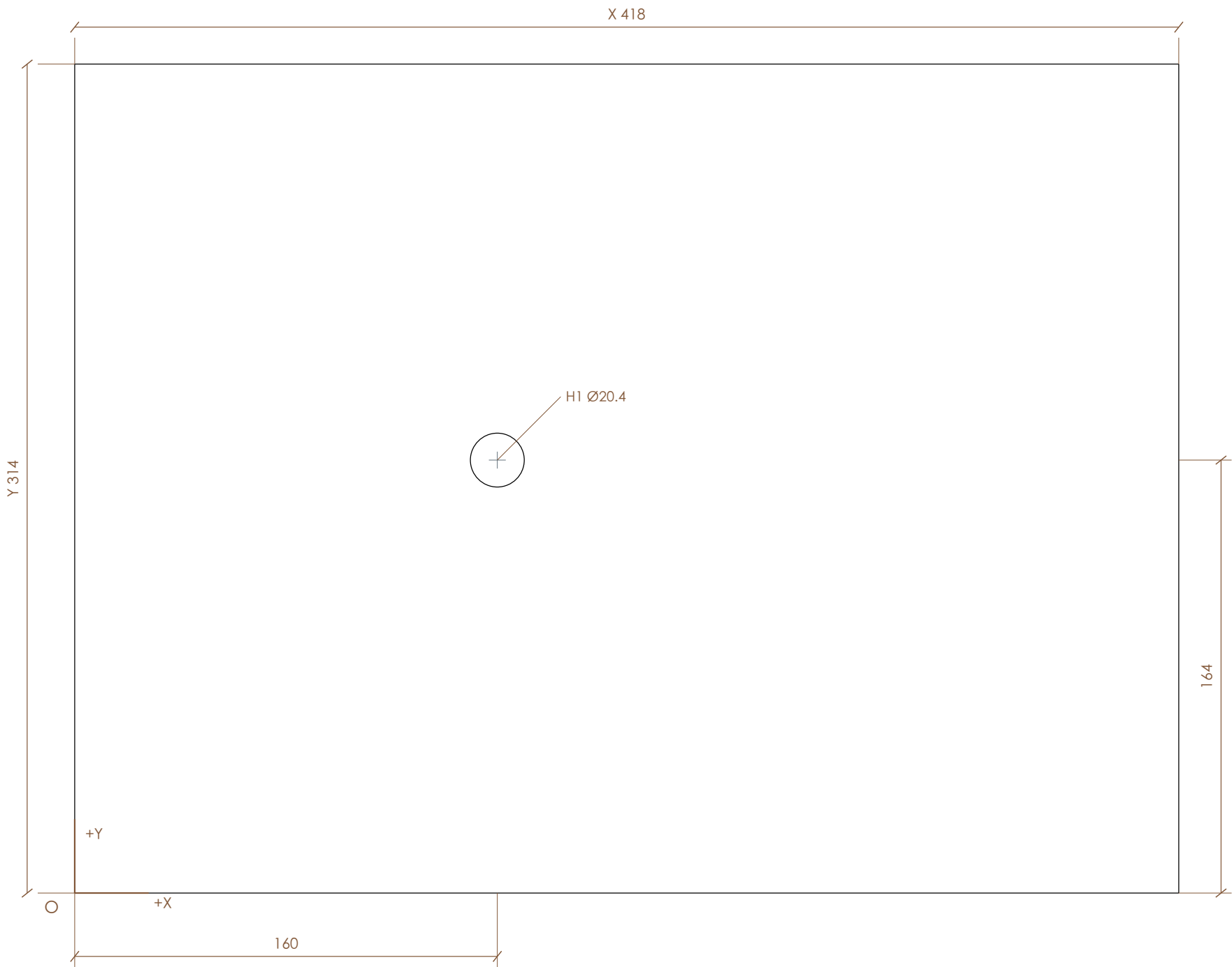
俯视 1:2 / 板厚 6
