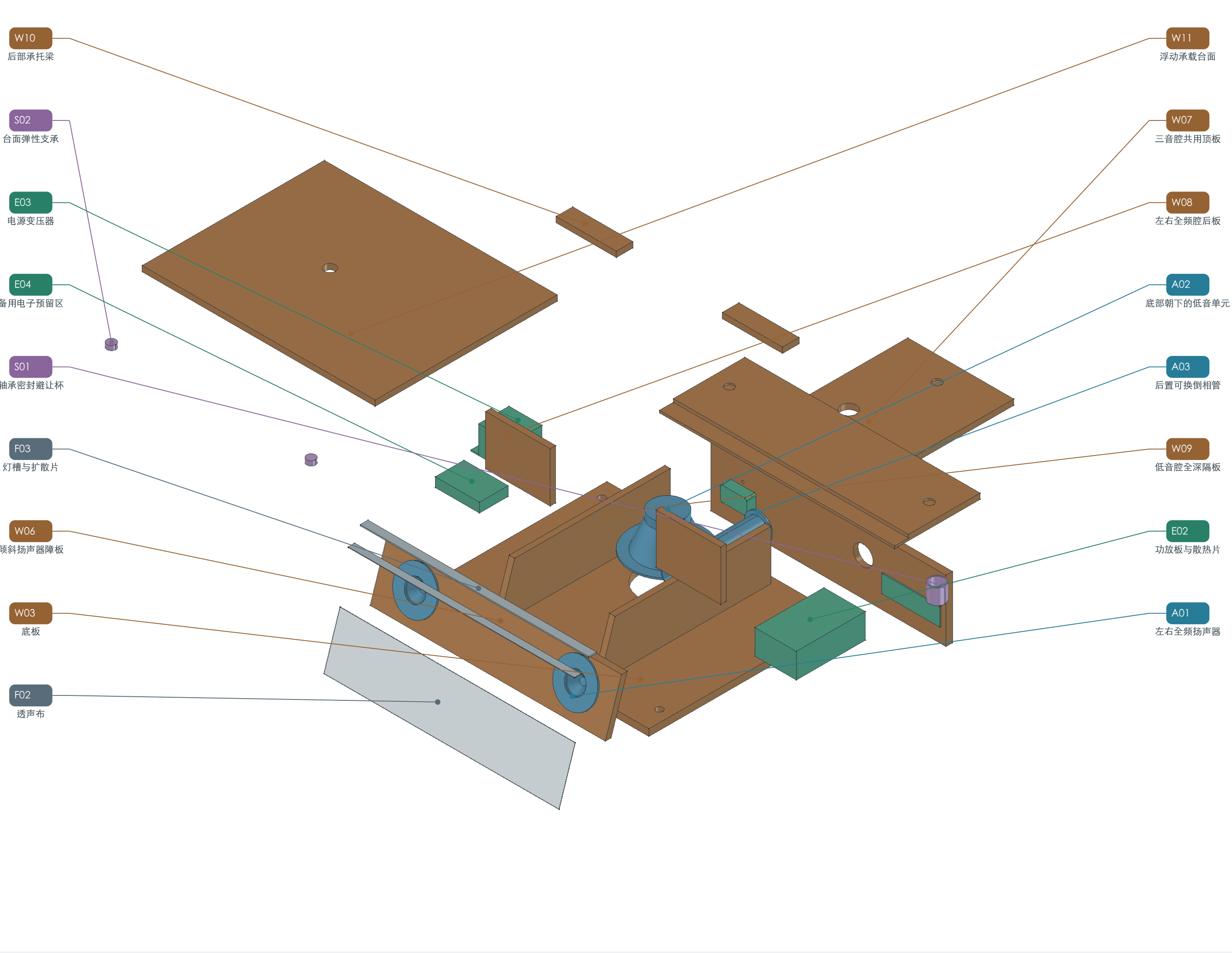
后部接口定位（后板半透明）
