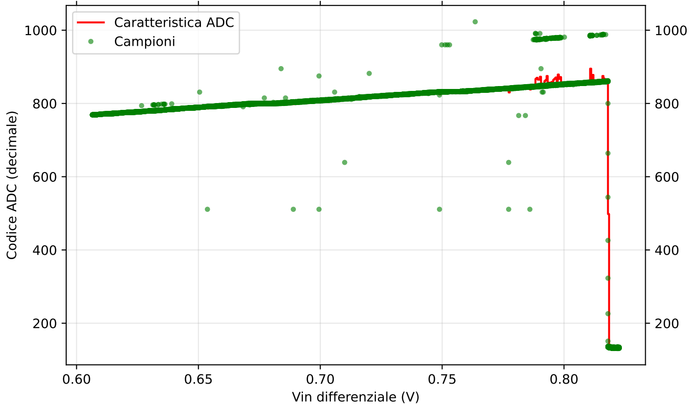
Caratteristica di Trasferimento ADC
