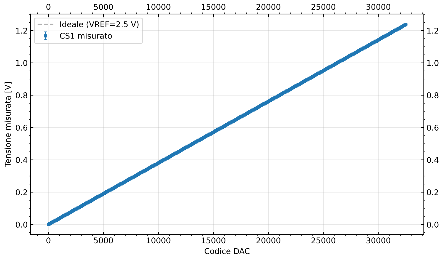
Caratteristica DAC -- CS1
