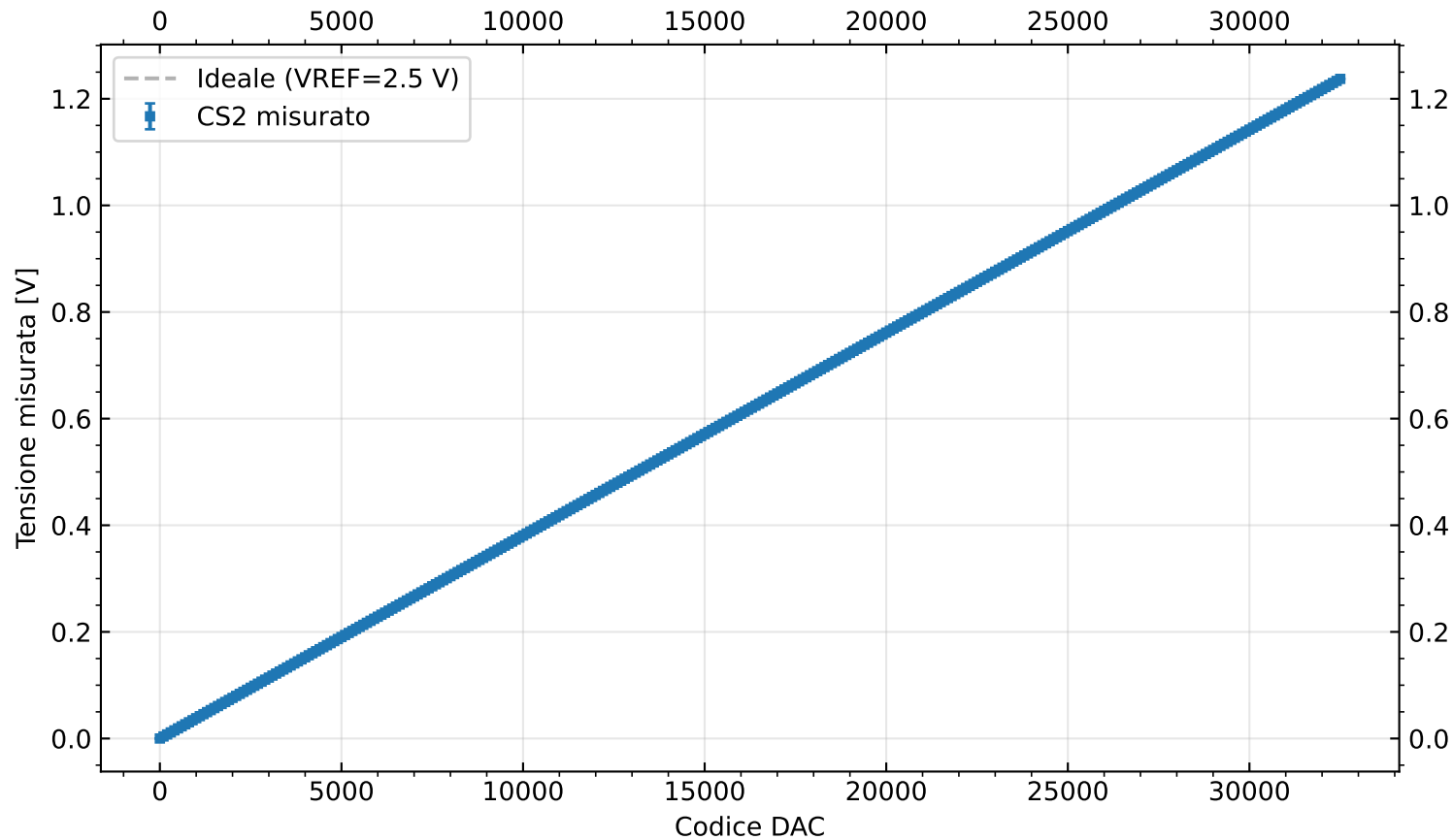
Caratteristica DAC -- CS2
