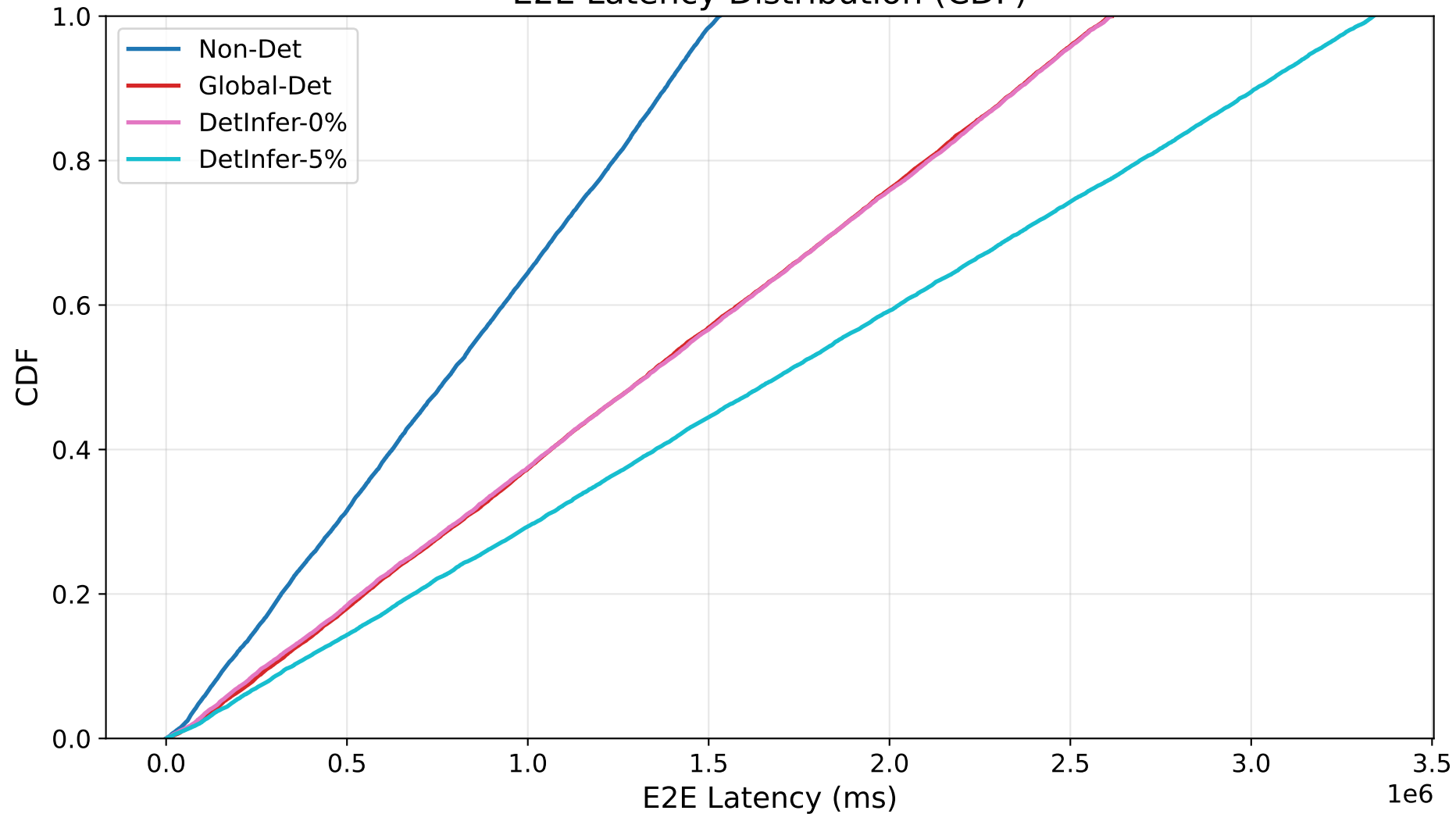
E2E Latency Distribution (CDF)
