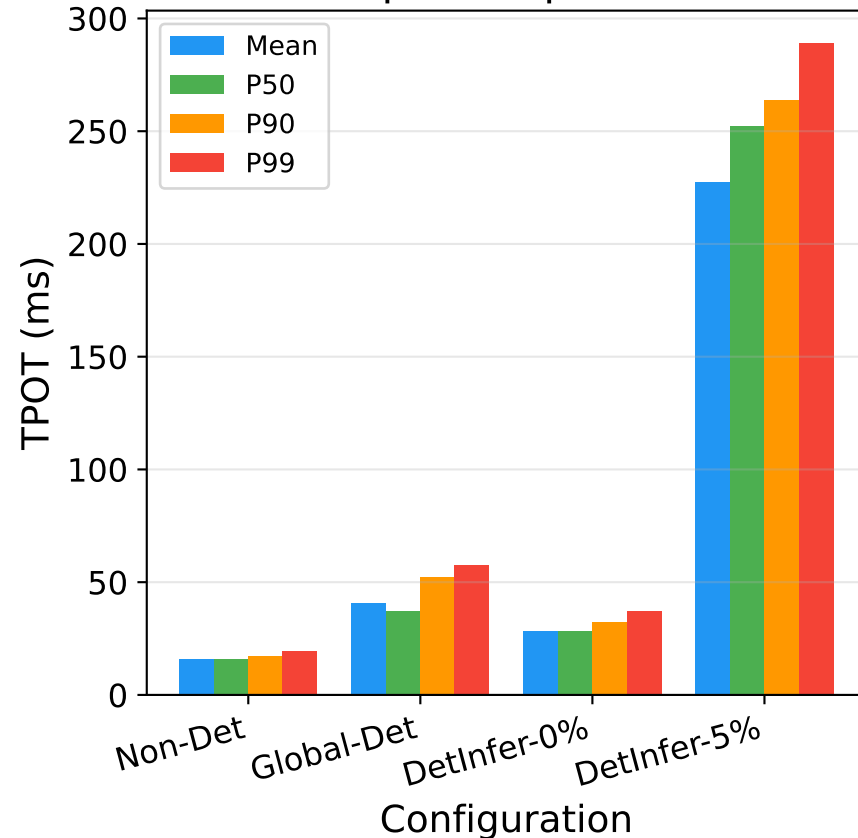
Time per Output Token
