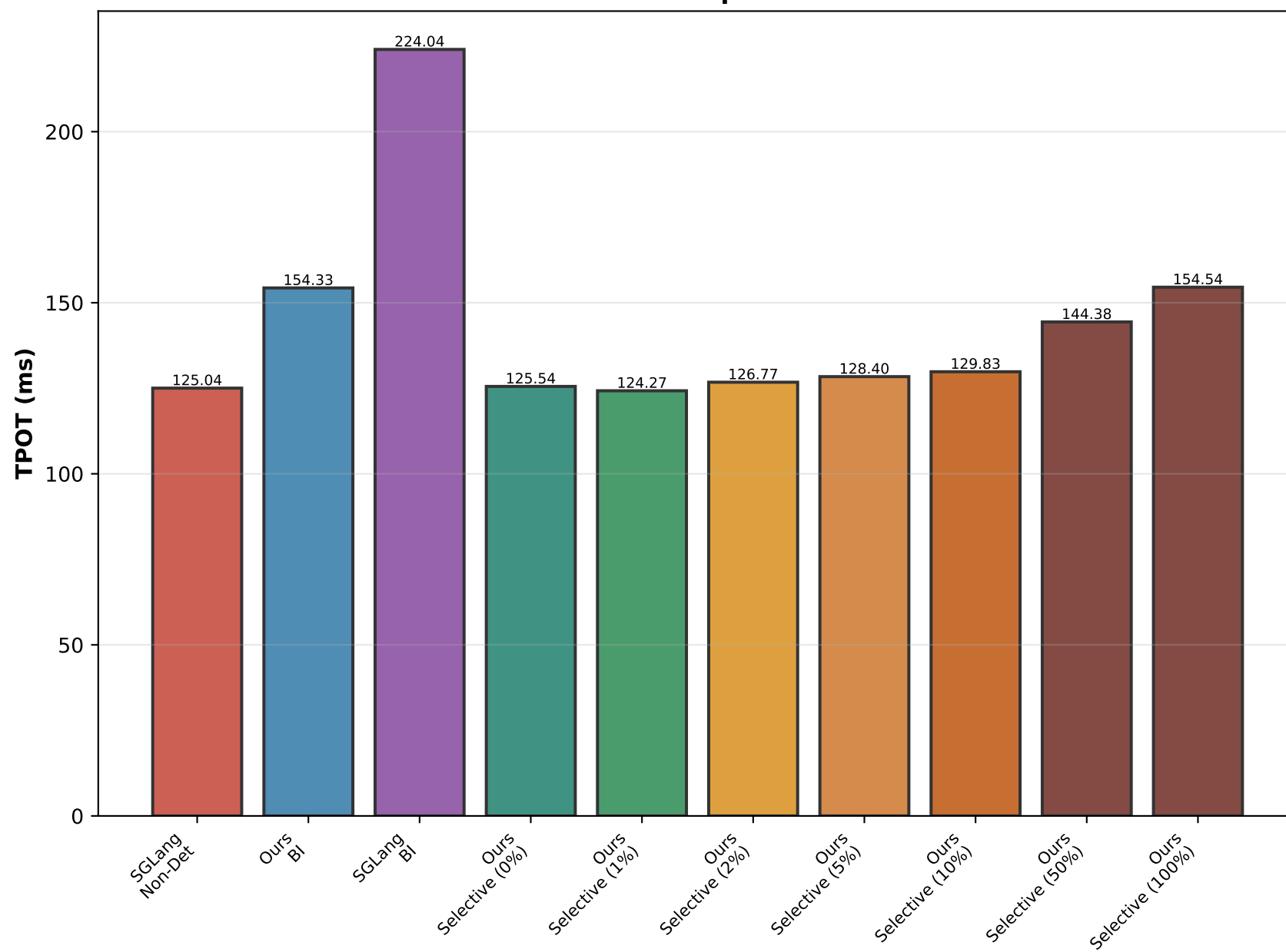
Time Per Output Token
