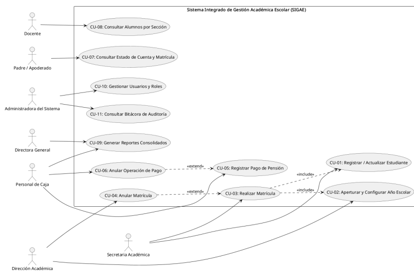
Figura 3: Modelo de casos de uso del sistema SIGAE.
