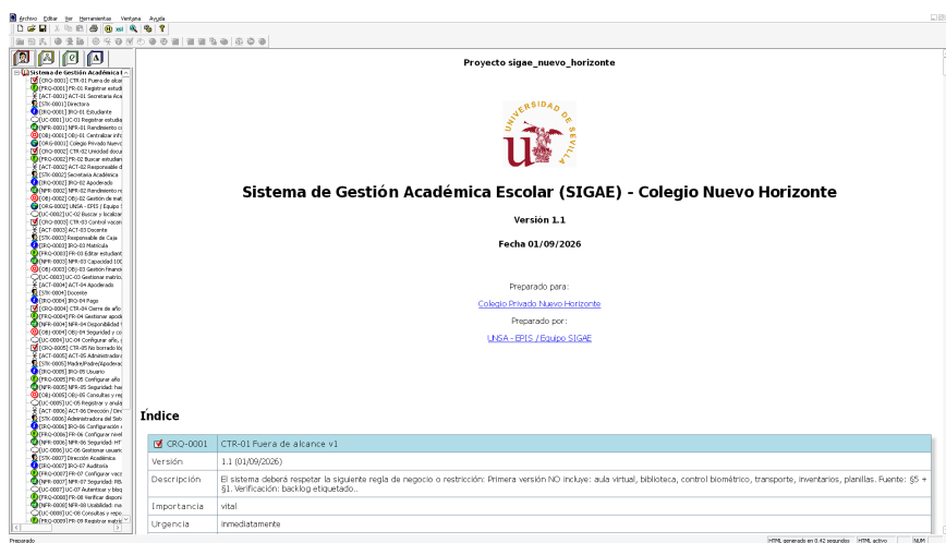
Figura 1: Captura de pantalla de la herramienta REM durante el modelado de requisitos.
