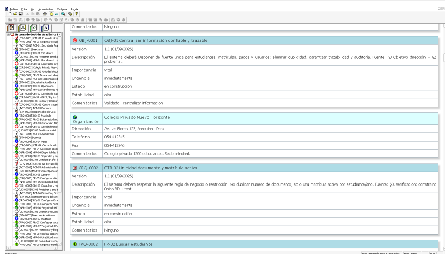
Figura 2: Panel de validación de consistencia y gestión de entidades en REM.
