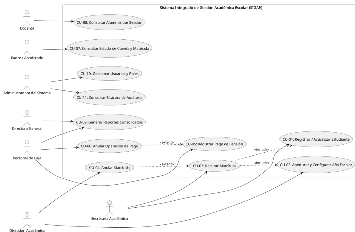
Figura 1: Modelo de casos de uso SIGAE. Actores: Secretaría, Caja, Docente, Apoderado, Administración y Dirección.
