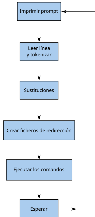
Figura 2.4: Pasos que realiza una shell interactiva
