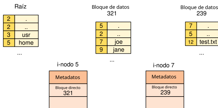
Figura 4.6: Ejemplo para resolver una ruta en Unix.
