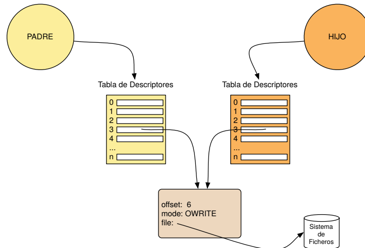
Figura 4.15: Ficheros abiertos padre e hijo: el hijo tiene su propia tabla, que apuntará a estructuras compartidas con el padre en el caso de los ficheros que ya estaban abiertos cuando se llamó a fork .
