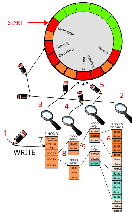
Figura 4.12: Detalle de los pasos de actualización del journal (datos y metadatos) por una escritura en un fichero.
