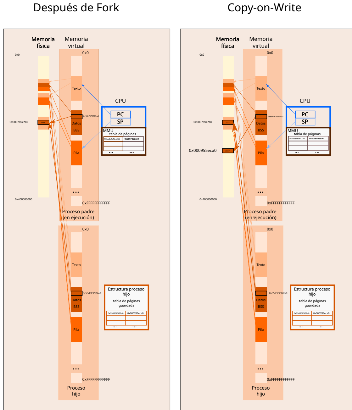
Figura 5.18: Cuando una página se modifica, su marco se duplica y se instala una nueva traducción.
