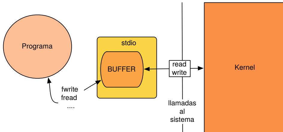
Figura 4.16: Stdio gestiona el buffer interno y sirve las peticiones desde el mismo.
