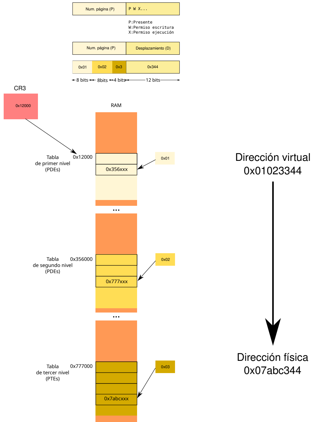
Figura 5.15: Ejemplo de traducción multinivel.
