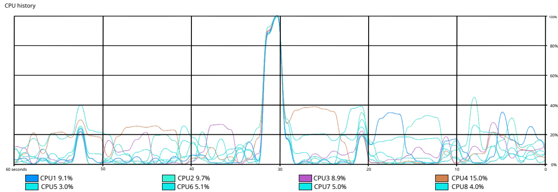
Figura 7.6: El programa con spin locks crea un pico de uso de todas las CPUs durante su ejecución; el programa que utiliza mutex , que ejecuta después, no genera un pico.
