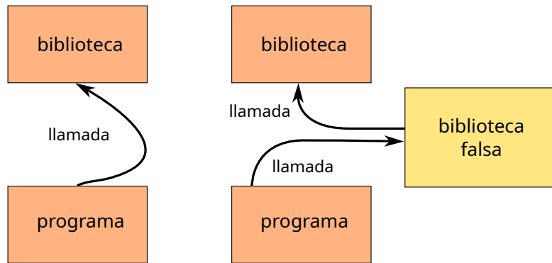
Figura 8.4: A la izquierda, una llamada a biblioteca normal. A la derecha, una biblioteca interpuesta (hooking).
