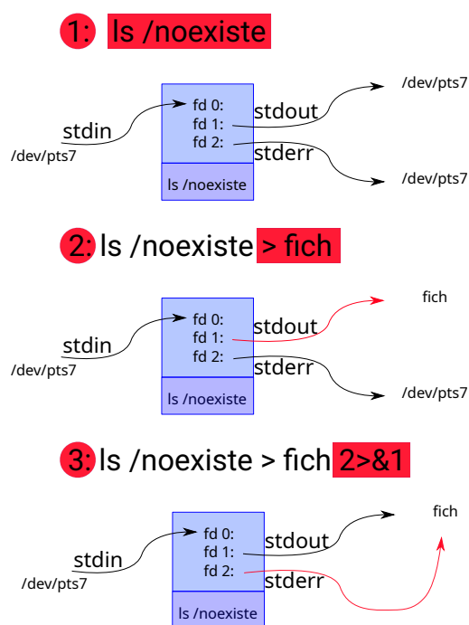
Figura 2.8: Redirección al fichero fich de la salida estándar y la salida de errores, ilustrado en tres pasos.
