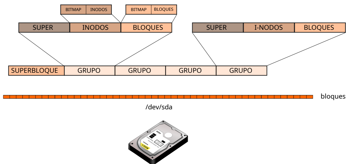
Figura 4.7: Áreas del disco en ext4
