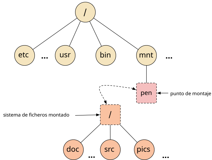
Figura 4.14: Ejemplo de espacio de nombres con dos sistemas de ficheros, el del raíz y otro montado de un pendrive.
