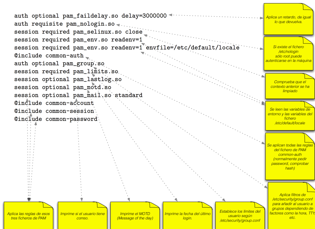
Figura 8.1: Ejemplo de un fichero de configuración de PAM para autenticar una aplicación.
