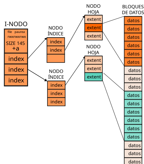
Figura 4.8: Extents en el ext4
