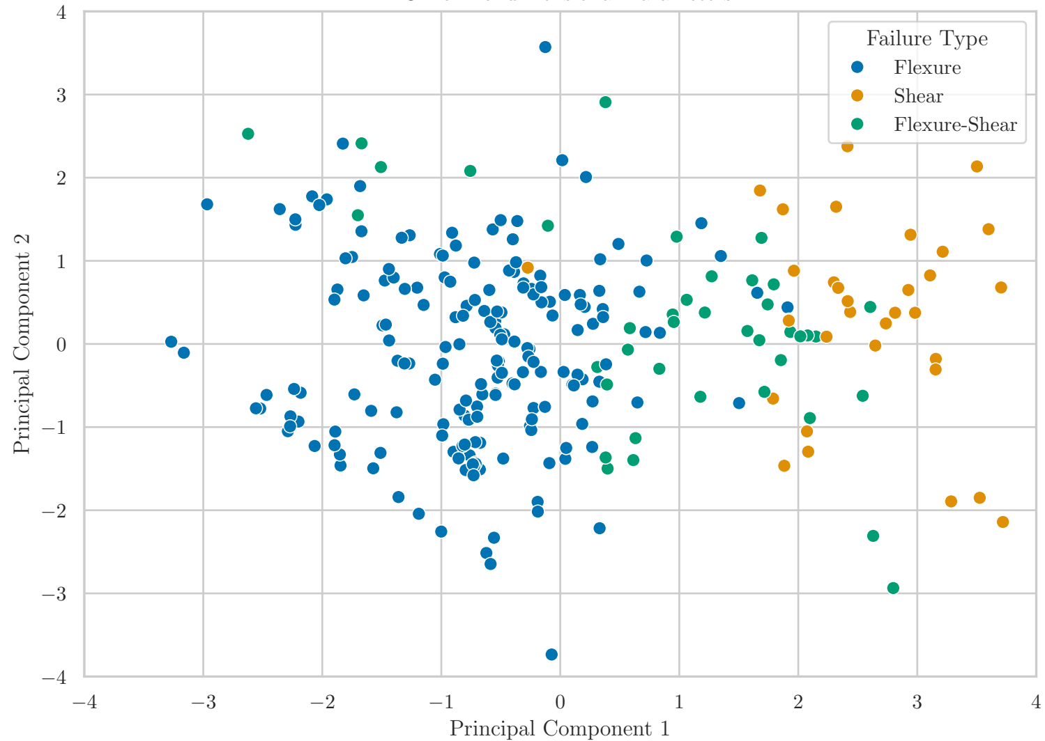
PCA of Nondimensional Parameters
