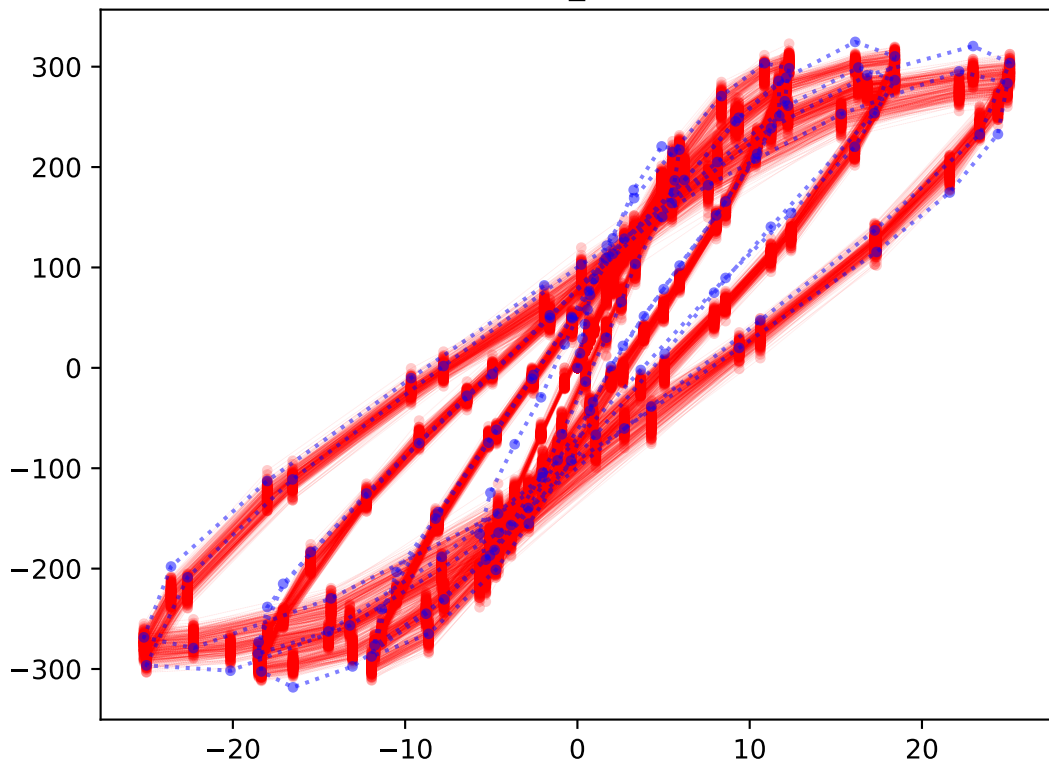
test_014
