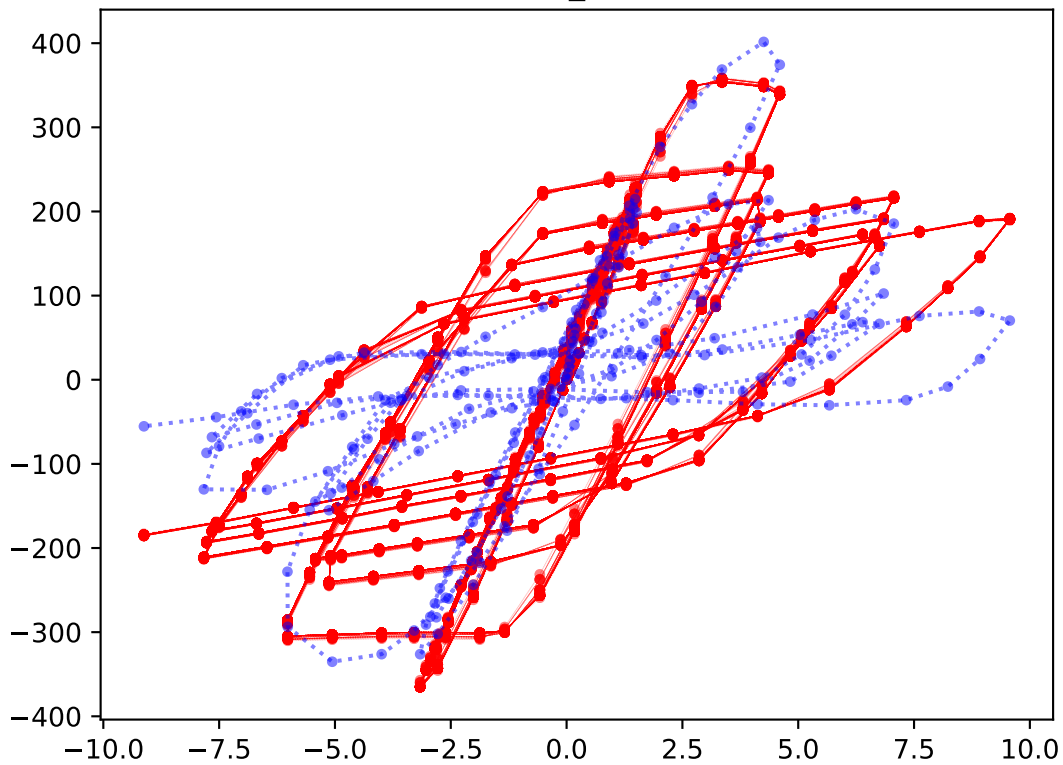
test_100
