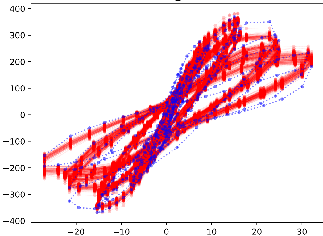
test_141
