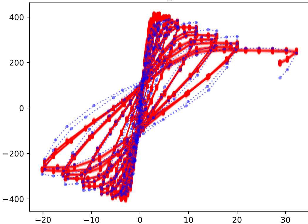
test_154
