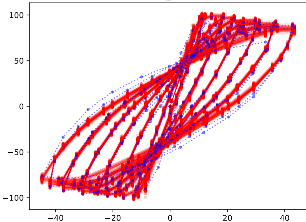
test_178
