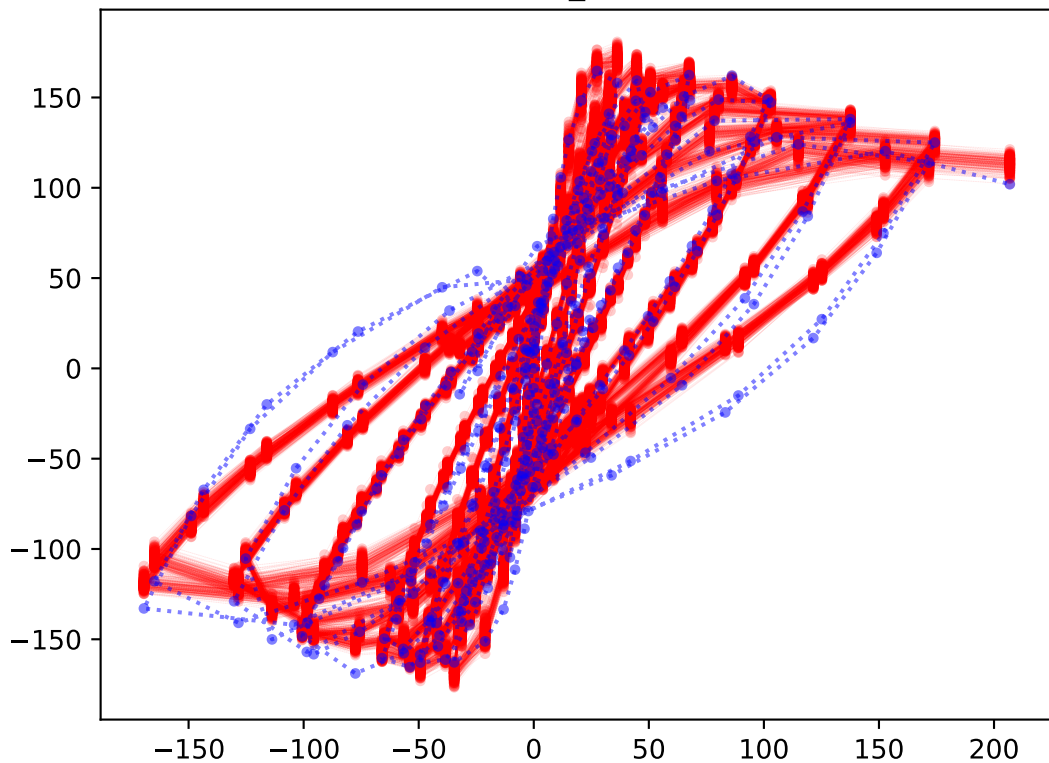
test_221
