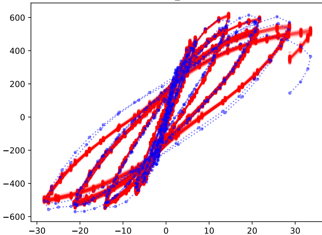
test_298
