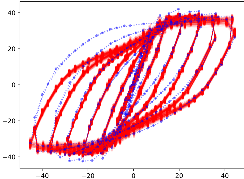
test_305
