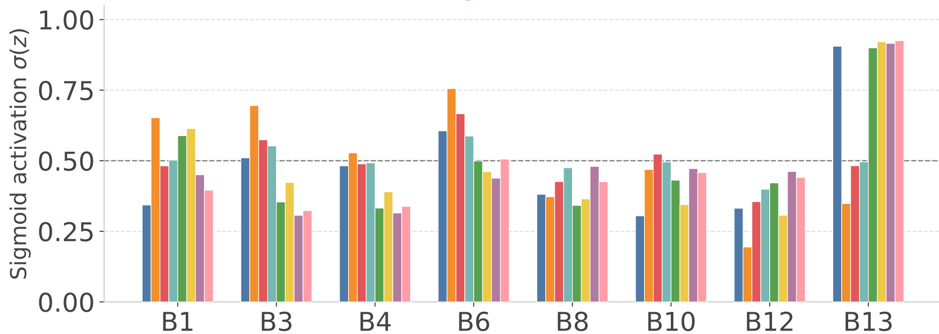
Bimerons (N=300)
