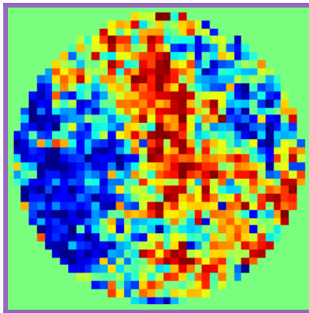
Bimerons
