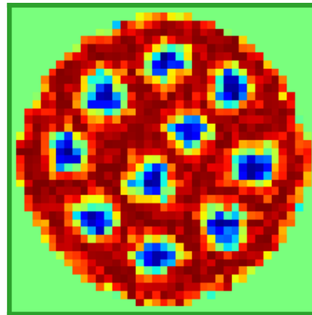
Skyrmions
