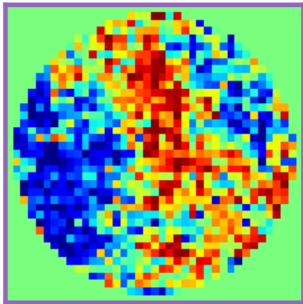
Bimerons
