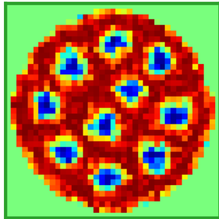
Skyrmions
