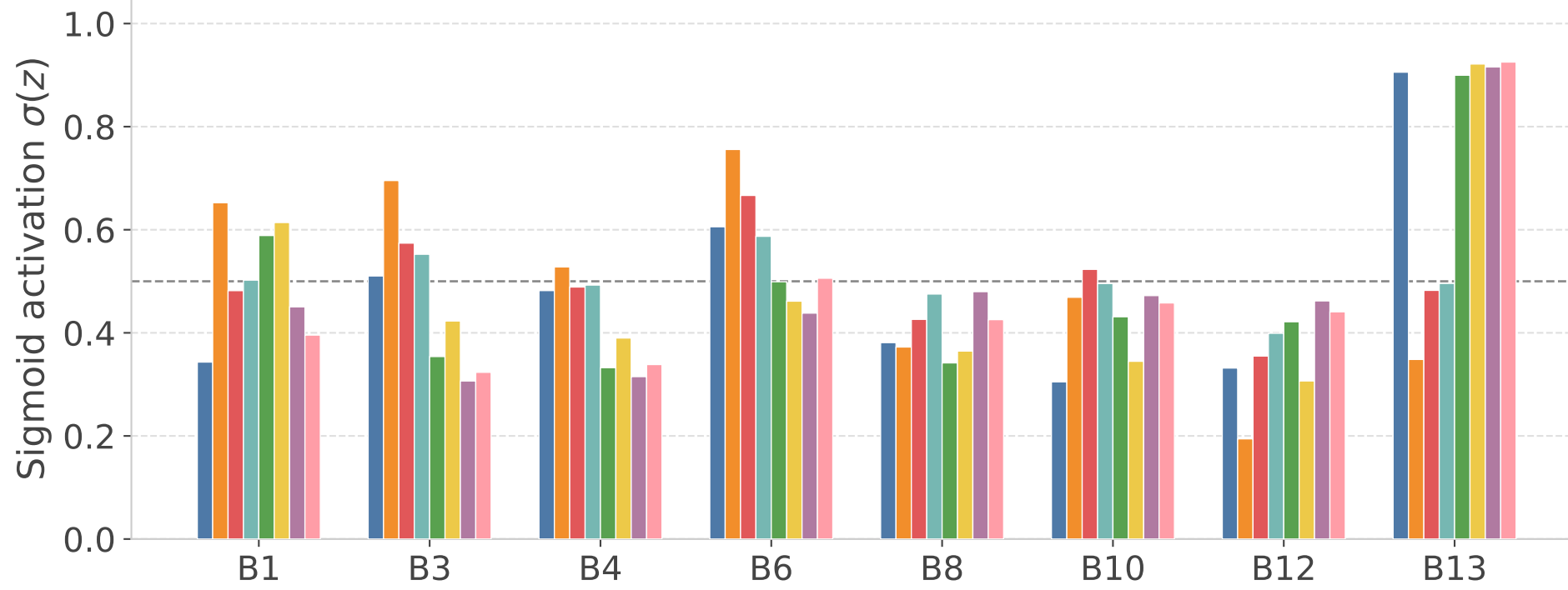
Bimerons (N=300)
