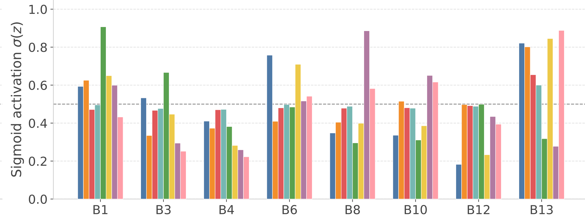
Skyrmions (N=300)
