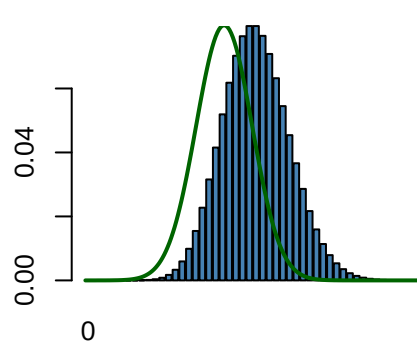
Sí aprox: \lambda=25 \rightarrow forma campana
