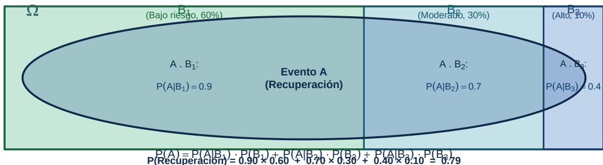
Teorema de la Probabilidad Total – Partición de \Omega y Evento A
