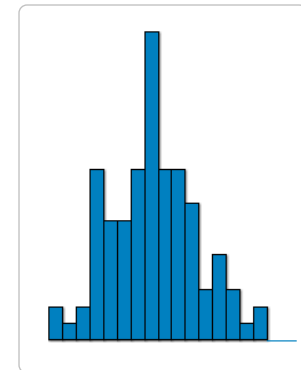
Estadísticos descriptivos
