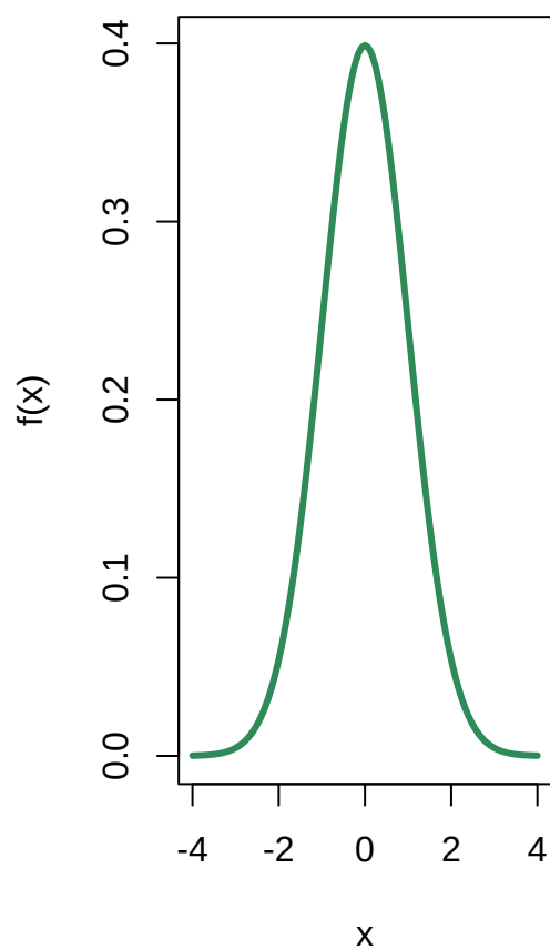
VA Continua: Normal(0,1)
