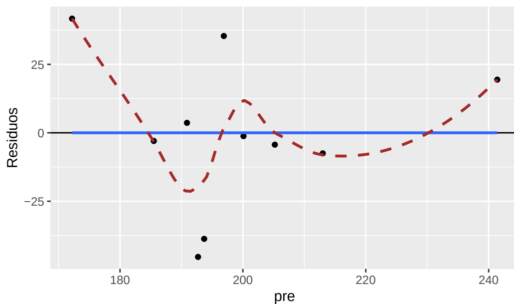
Distancias residuales respecto al modelo
