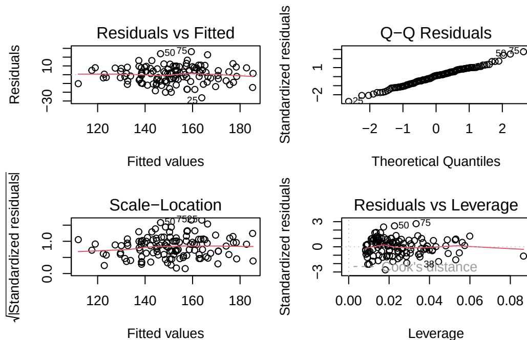
Figura 10.1: Gráficos de diagnóstico del modelo de regresión múltiple PAS \sim \text{Edad} + \text{IMC} . La distribución aleatoria de residuos y el ajuste al Q-Q plot validan los supuestos del modelo.
