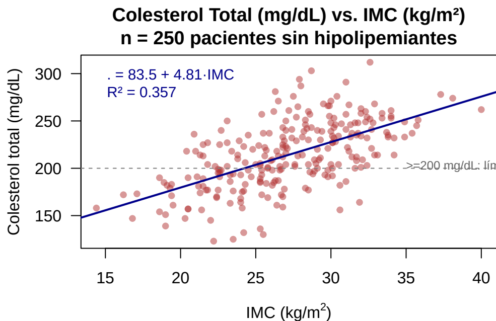
Figura 9.3: Regresión lineal Colesterol Total ~ IMC. Los 250 puntos representan pacientes sin tratamiento hipolipemiante. La línea muestra la relación estimada: por cada kg/m 2 adicional de IMC, el colesterol aumenta en promedio ~5 mg/dL.
