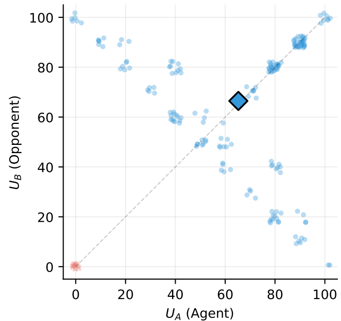
LA-GRPO All-Equal
