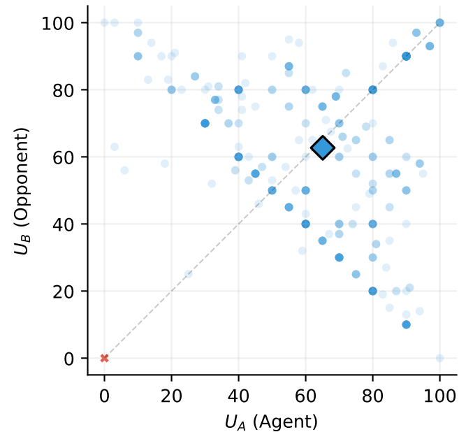
GRPO All-Equal
