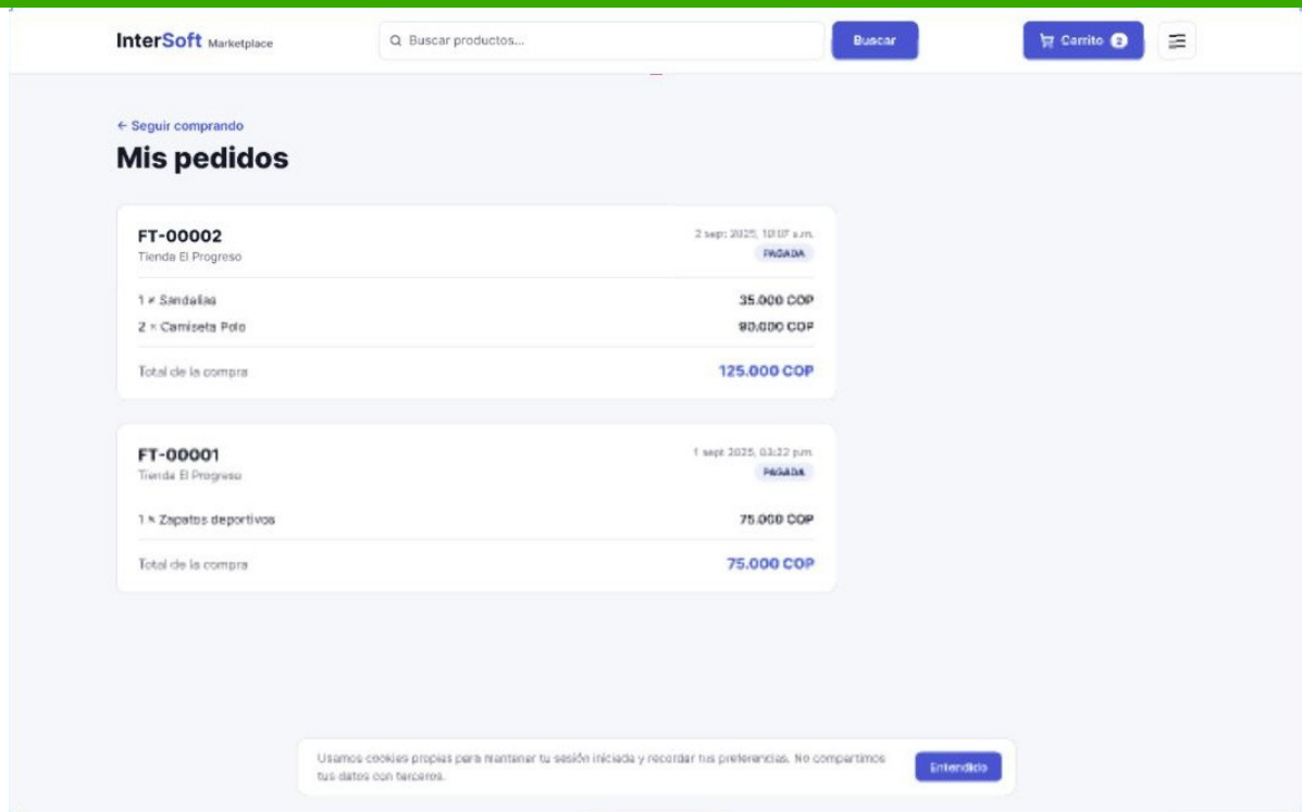
Figura 13. Vista mis-pedidos. Tarjetas de factura con número, establecimiento, fecha, estado, líneas de detalle y total.
