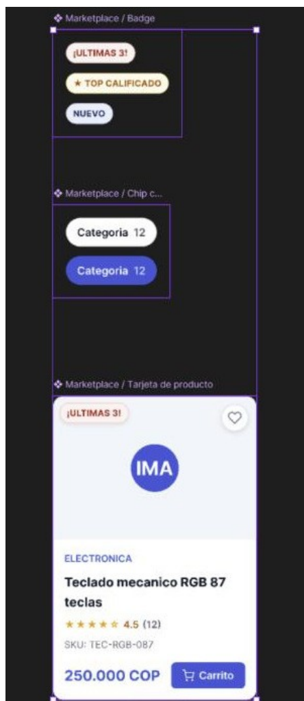
Figura 7. Los tres componentes del sistema: conjunto Badge con sus tres variantes, conjunto Chip categoría con dos estados y el componente Tarjeta de producto.
