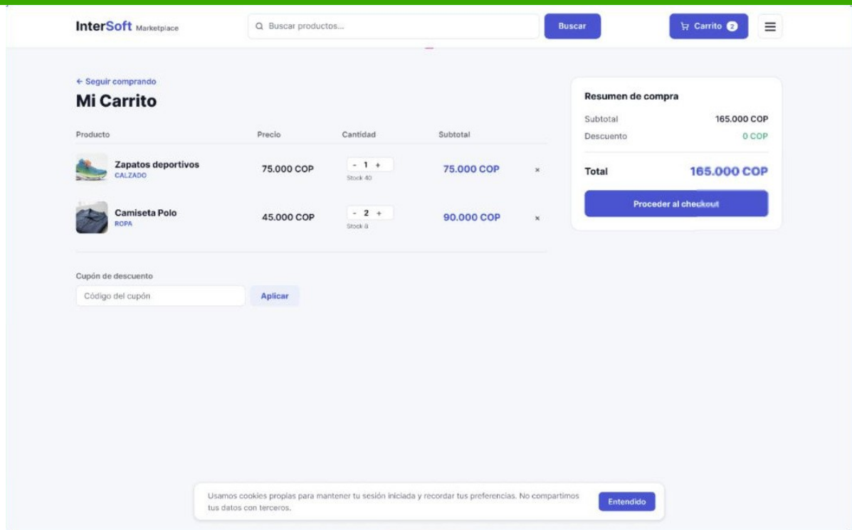
Figura 11. Vista mi-carrito. Tabla de productos con control de cantidades, campo de cupón y panel de resumen de compra.
