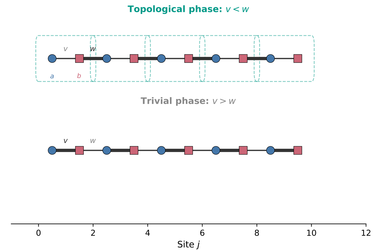
(d) SSH dimer model
