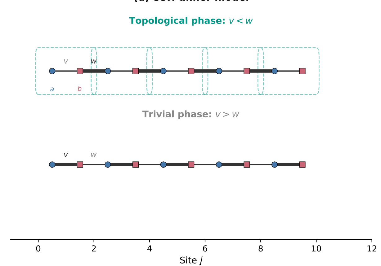
(d) SSH dimer model
