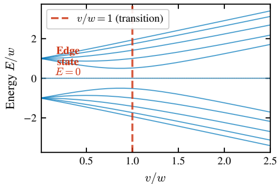
(d) SSH dimer model
