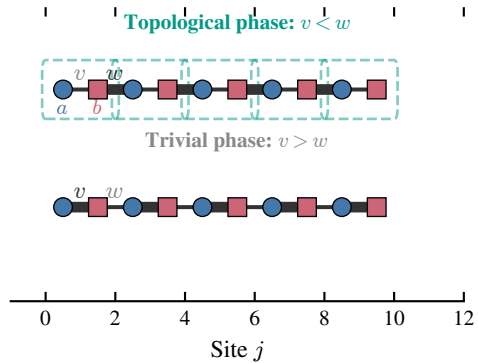
(d) SSH dimer model
