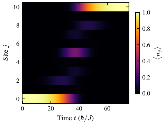
(d) STA global \sin^2 : t_{tr}=75.0 , f=1.0000
