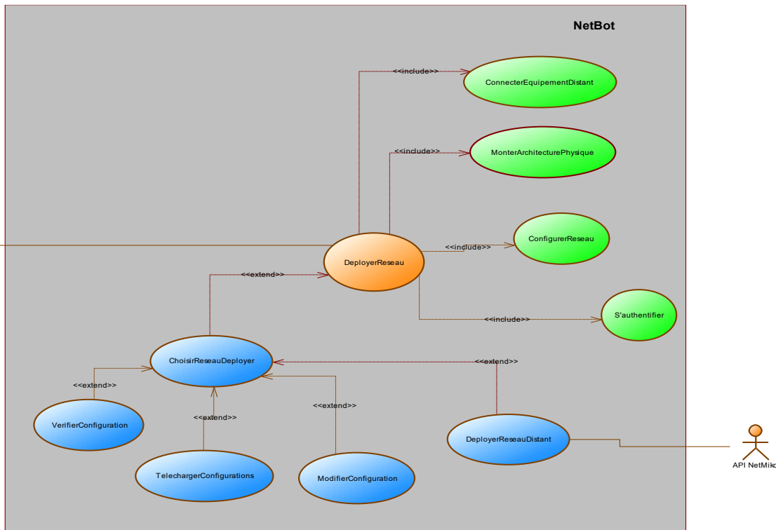
Figure 8 diagramme de cas d'utilisation spécifique déployé réseau
