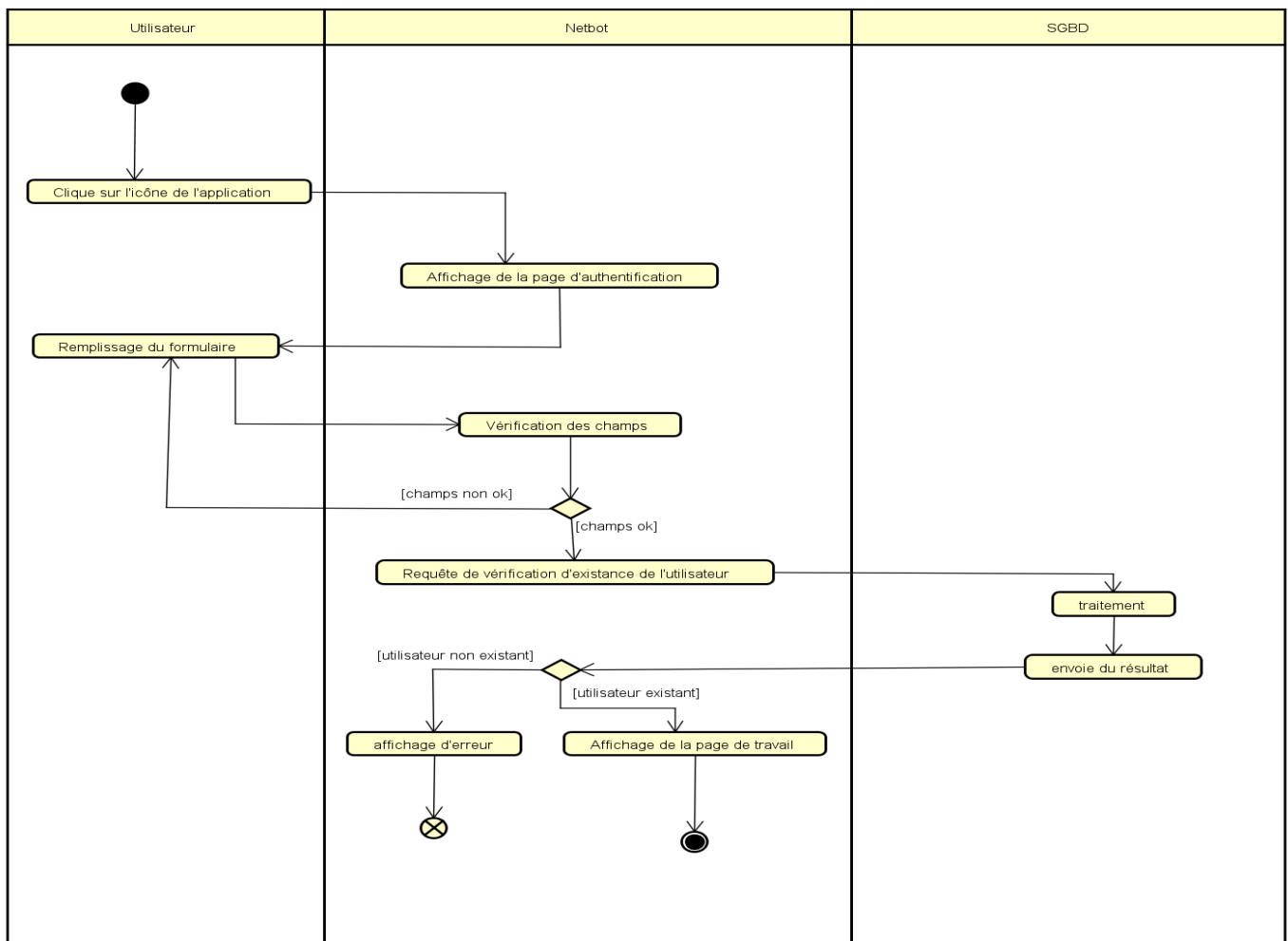
Figure 19 diagramme d'activité du cas s'authentifier
