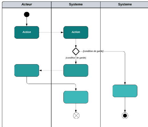
Figure 18 exemple de diagramme d'activité
