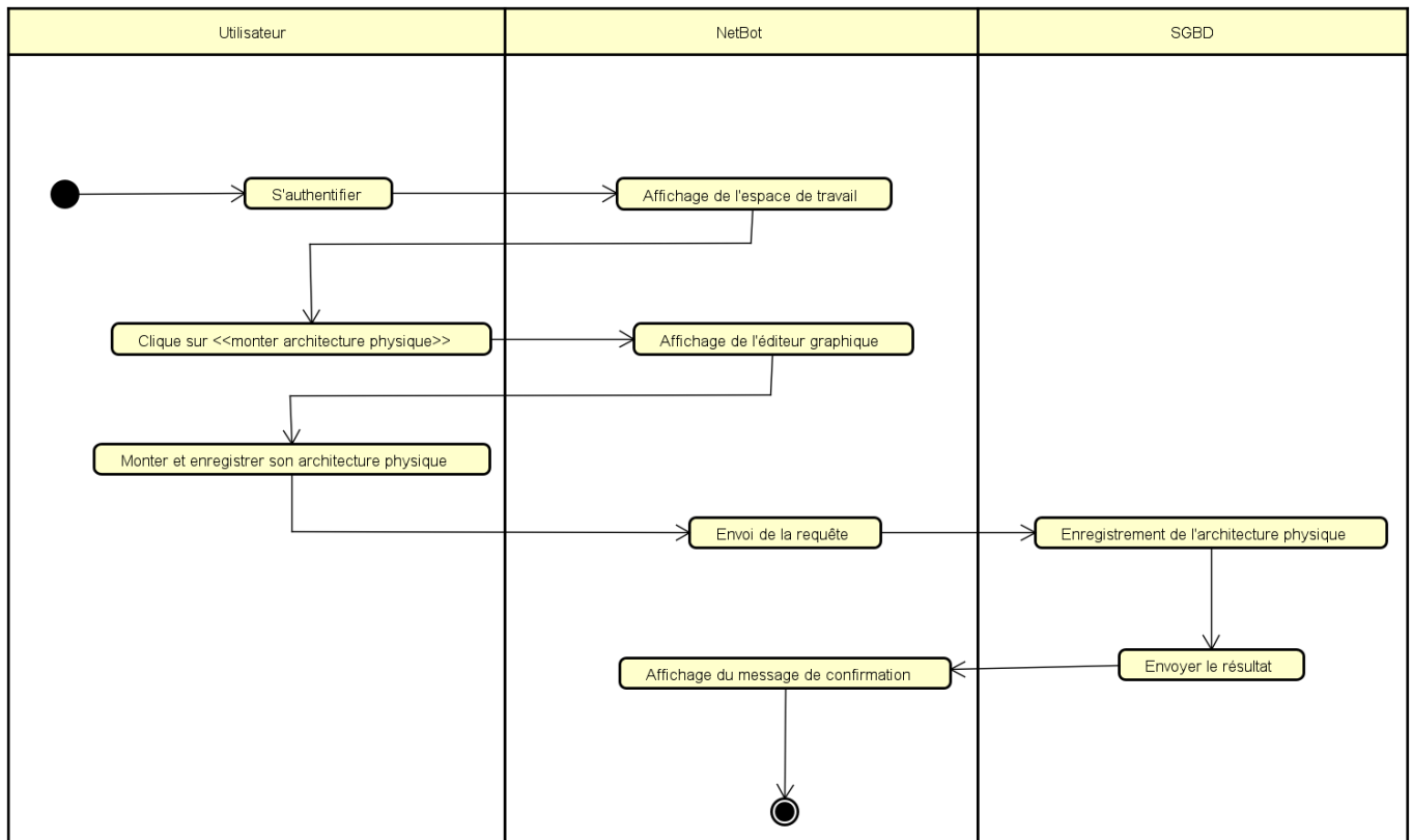
Figure 21 diagramme d'activité du cas monter architecture physique
