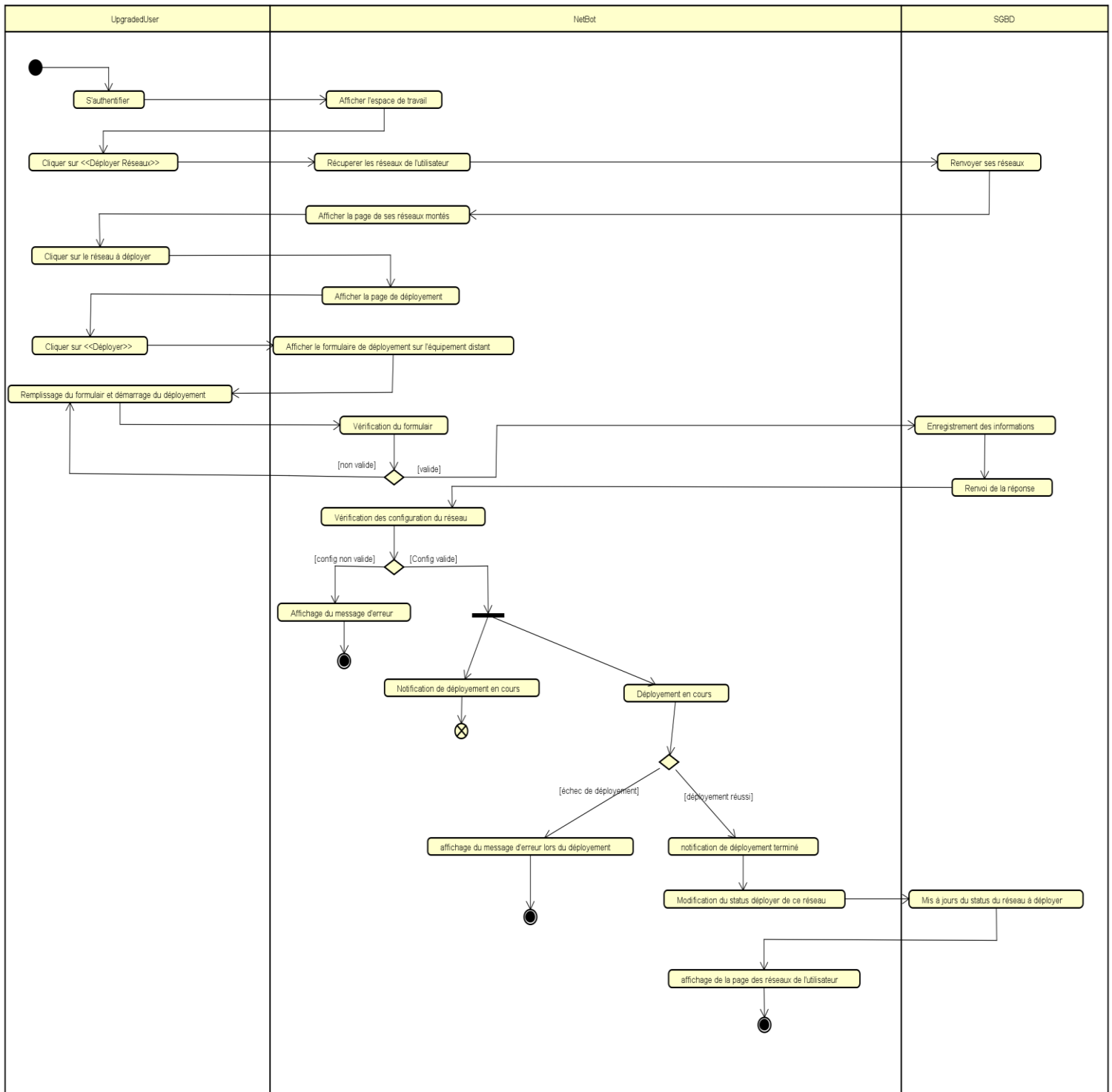
Figure 22 diagramme d'activité du cas déployé réseau
