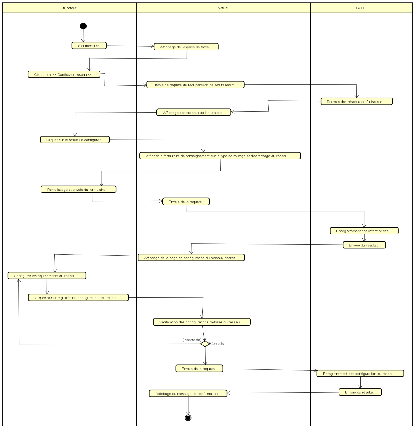
Figure 20 diagramme d'activité du cas configurer réseau
