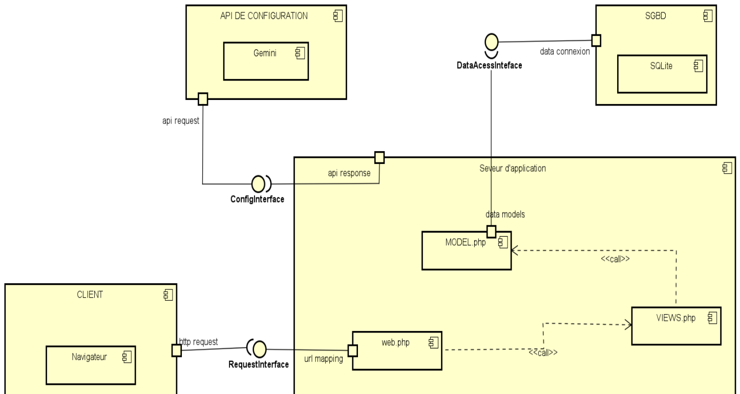
Figure 33 diagramme de composant de notre solution
