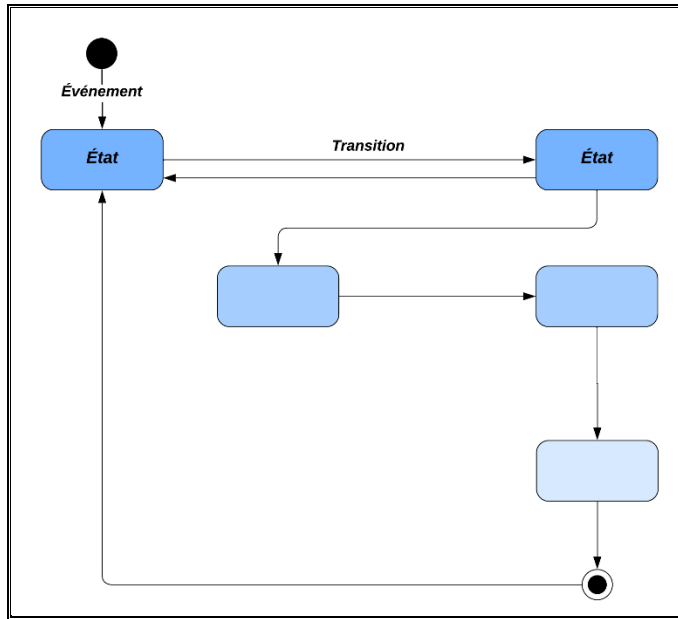
Figure 25 formalisme du diagramme d'état transition
