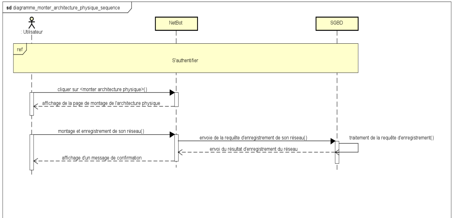
Figure 15 diagramme de séquence du cas d'utilisation monter architecture physique
