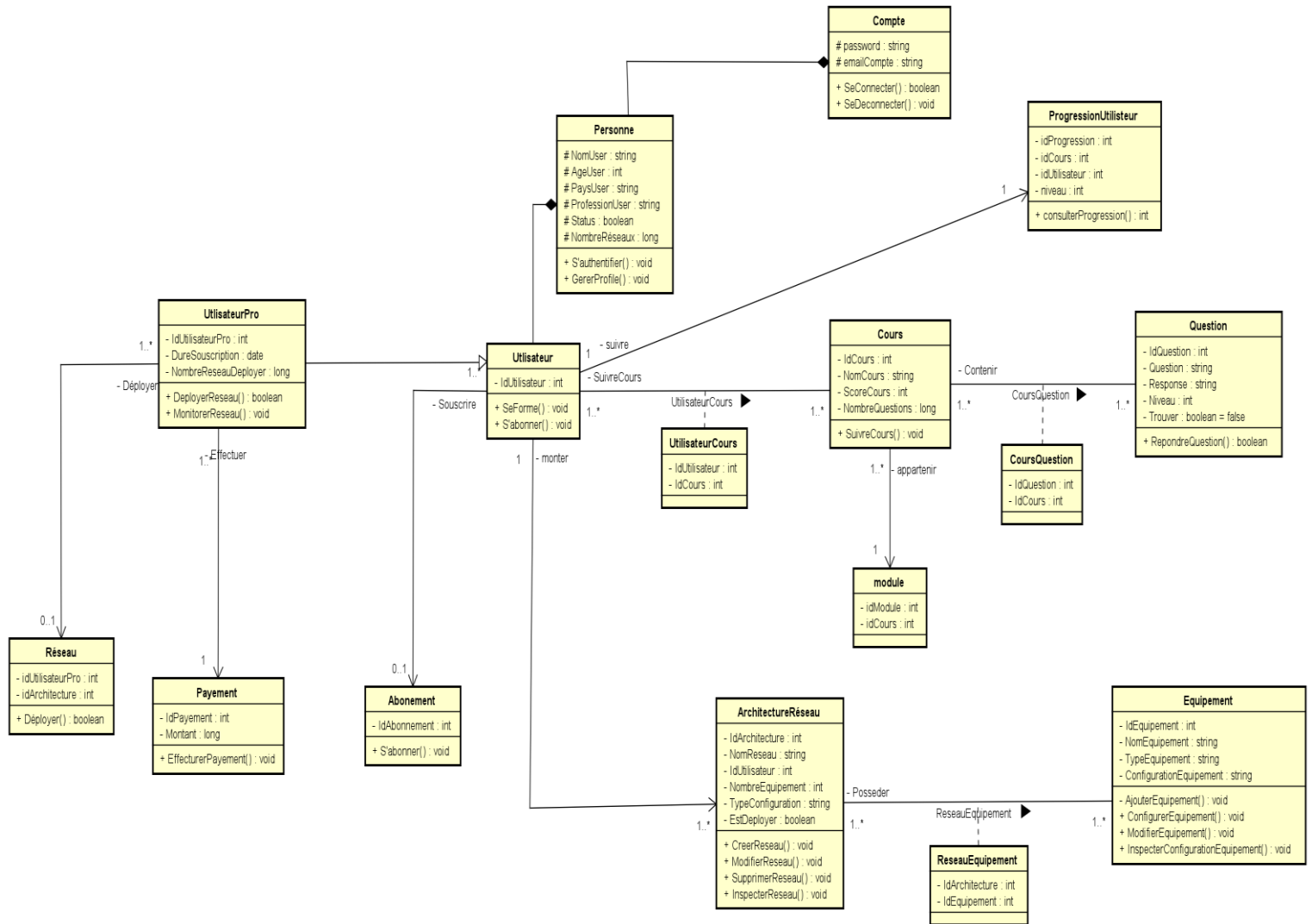
Figure 24 diagramme de classe de notre système
