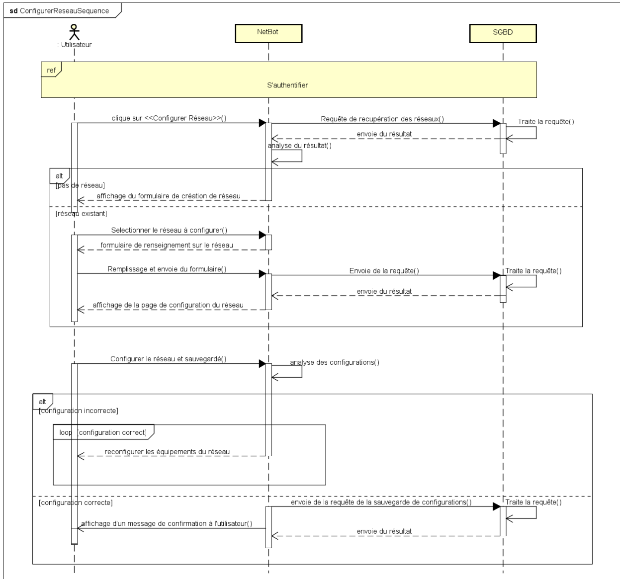
Figure 16 diagramme de séquence du cas configurer réseau
