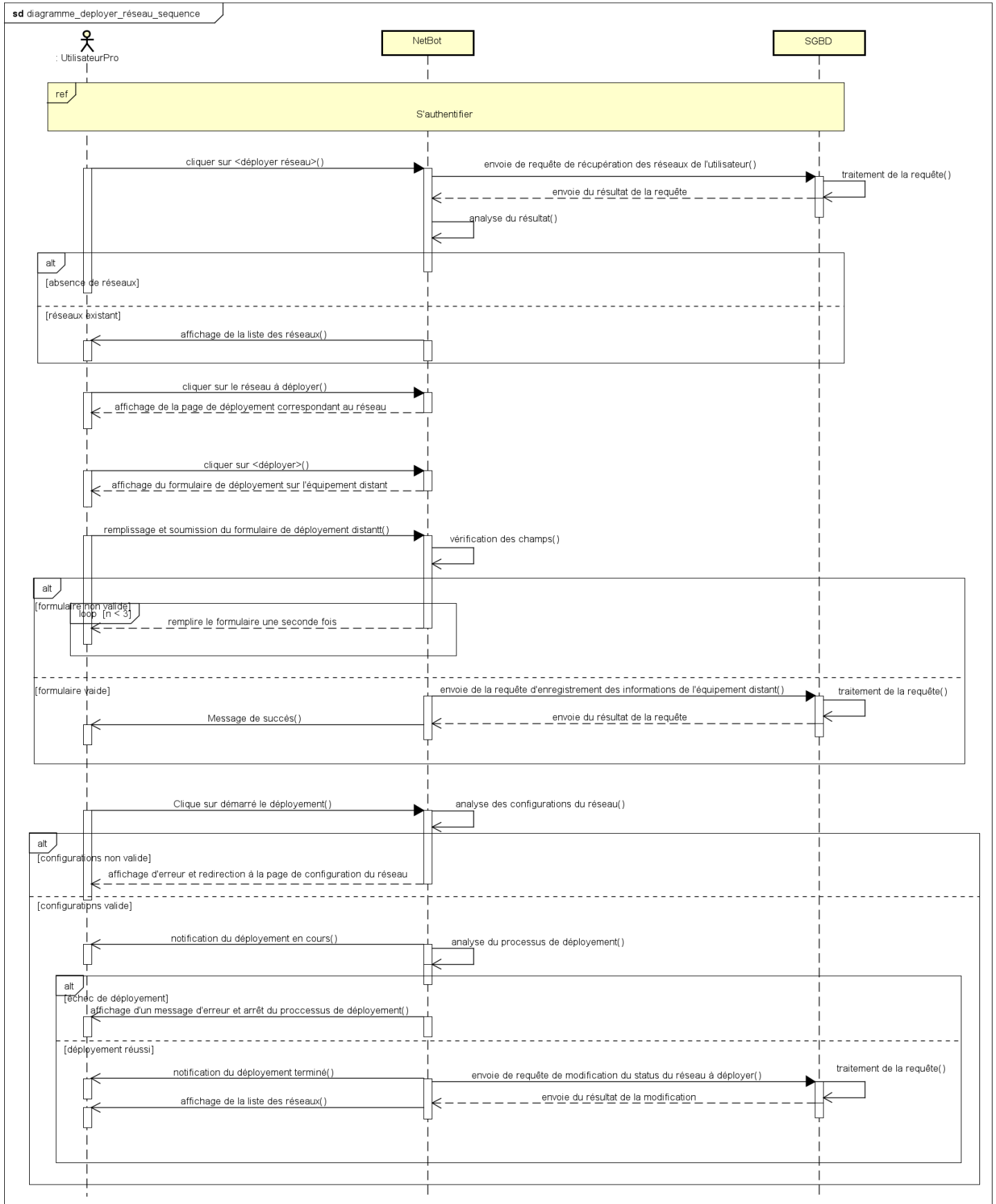
Figure 17 diagramme de séquence du cas déployé réseau
