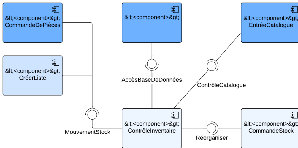
Figure 32 formalisme du diagramme de composant
