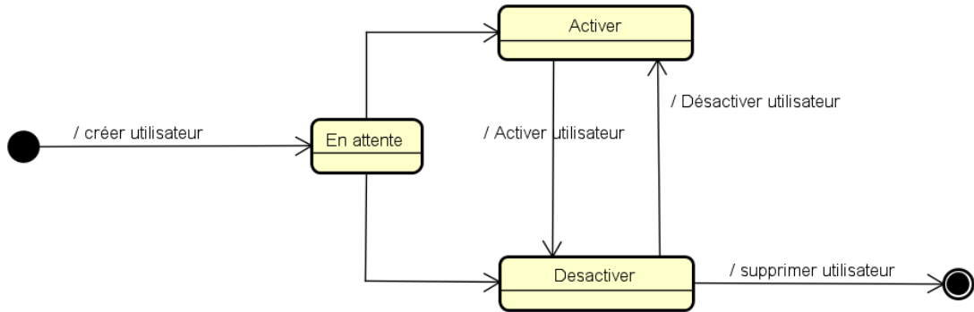
Figure 27 Diagramme d'état transition d'un utilisateur
