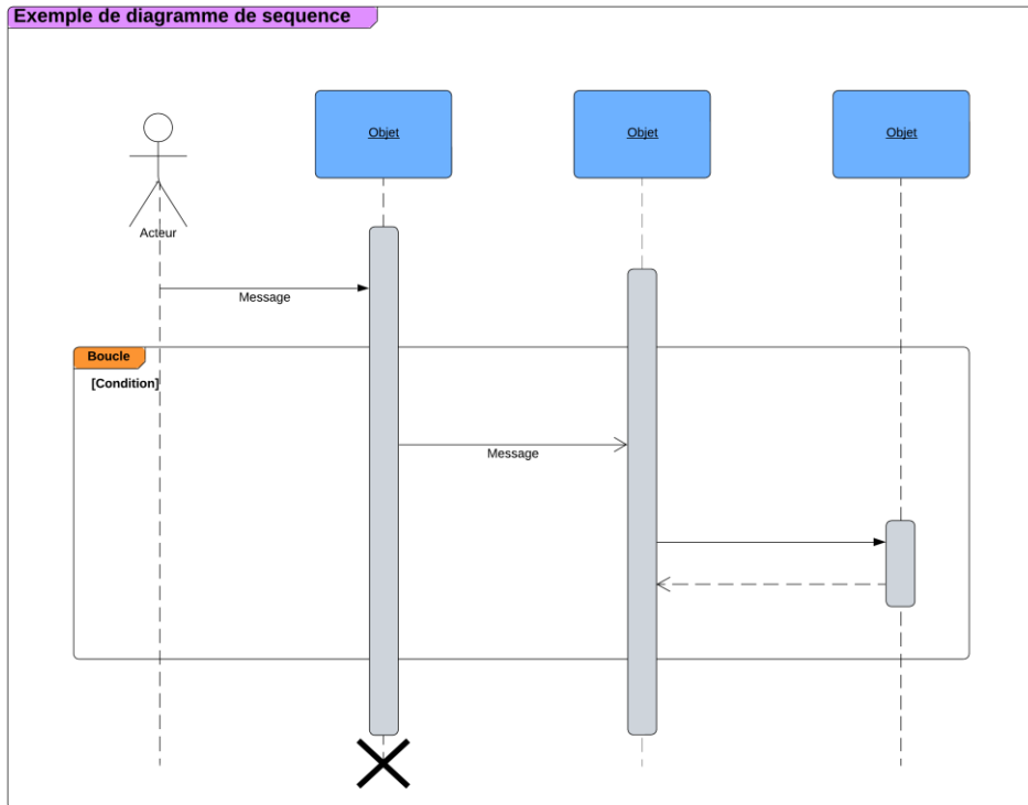
Figure 13 exemple de diagramme de séquence
