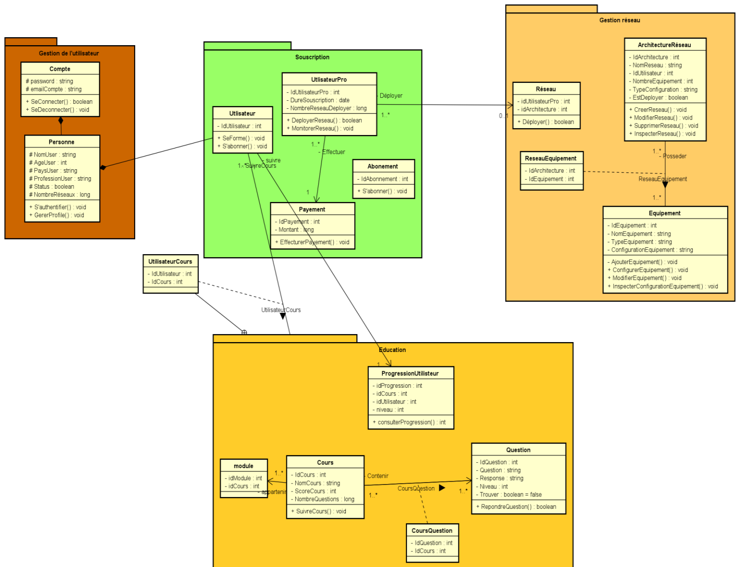
Figure 28 diagramme de paquetage de notre système
