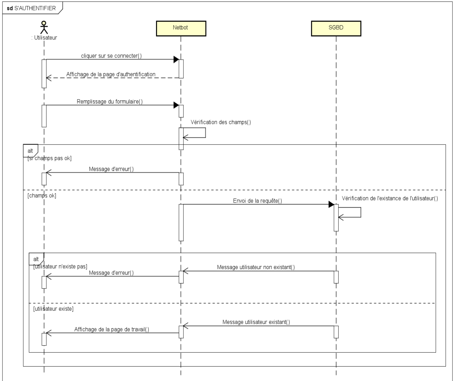
Figure 14 diagramme de séquence du cas s'authentifier
