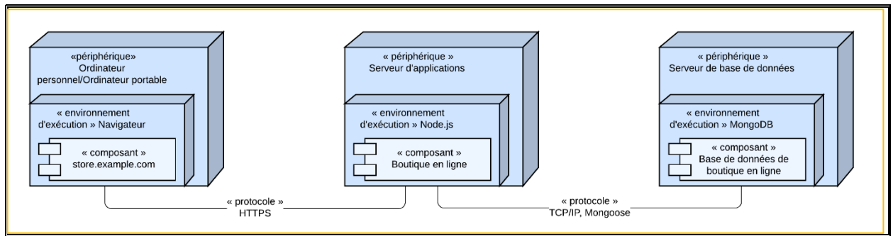
Figure 30 formalisme du diagramme de déploiement
