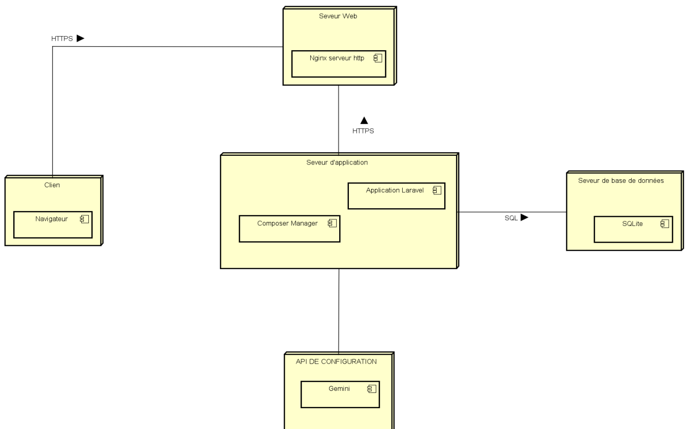
Figure 31 diagramme de déploiement de la solution
