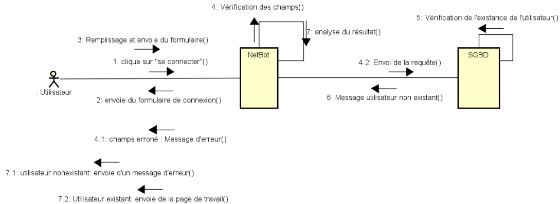
Figure 9 diagramme de communication du cas s'authentifier
