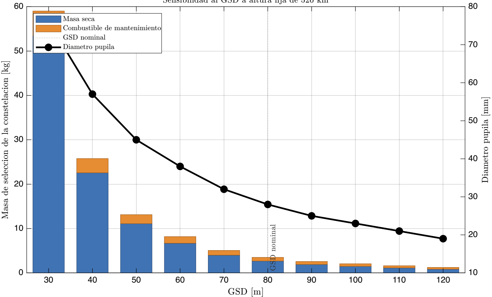
Sensibilidad al GSD a altura fija de 520 km
