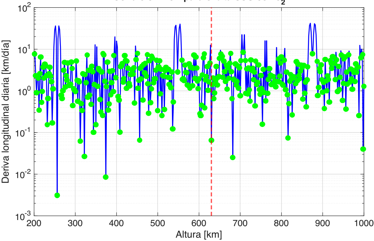
Condición RGT para órbita SSO con J_2
