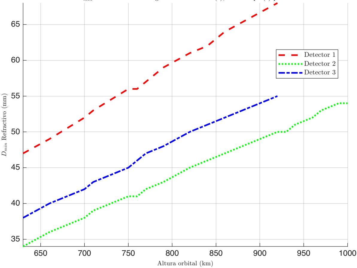
h vs D_{min} - Refractivo - Configuración: 2 satélite(s), 2 telescopio(s) por satélite
