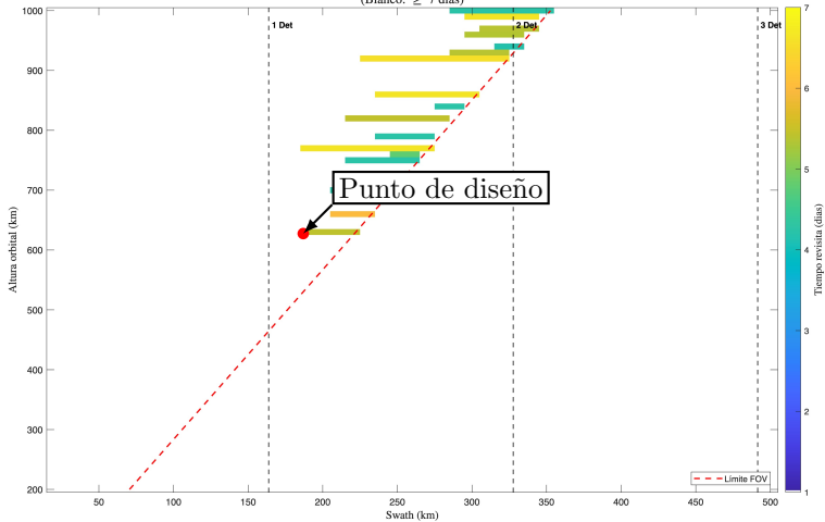
Tiempo Revisita - 2 Satelite(s); 2 Telescopio(s); Refractivo; Detector 2 (Blanco: \geq 7 dias)
