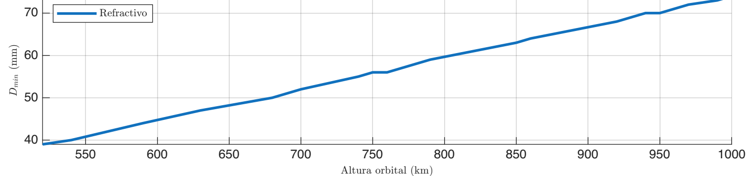
h vs D_{min} viable - Detector 2 - Configuración: 2 satélite(s), 2 telescopio(s) por satélite
