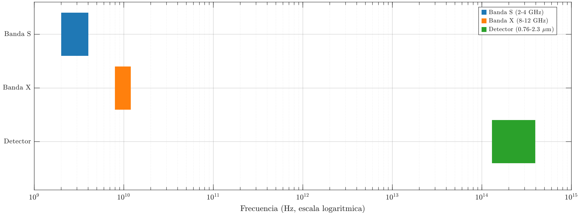
Ubicacion de las Bandas S, X y Detector en el Espectro de Frecuencias
