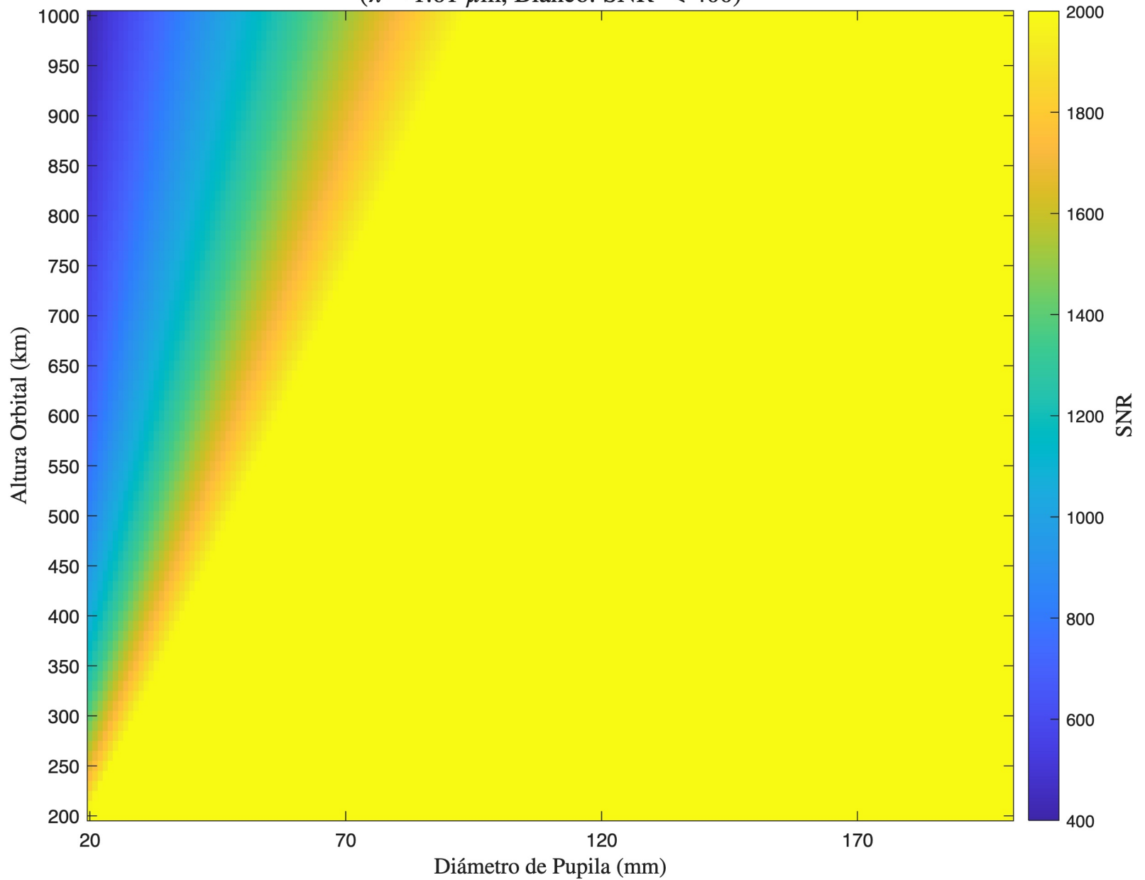
SNR - Refractivo - Detector 1 ( \lambda = 1.61 \mu\text{m} , Blanco: SNR < 400)
