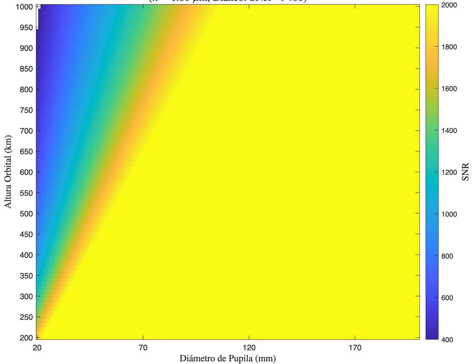
SNR - Korsch - Detector 1 ( \lambda = 1.61 \mu\text{m} , Blanco: SNR < 400)
