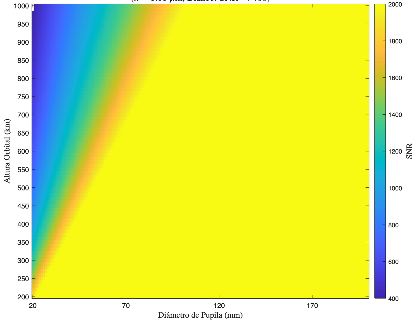
SNR - Cassegrain - Detector 1 ( \lambda = 1.61 \mu\text{m} , Blanco: SNR < 400)
