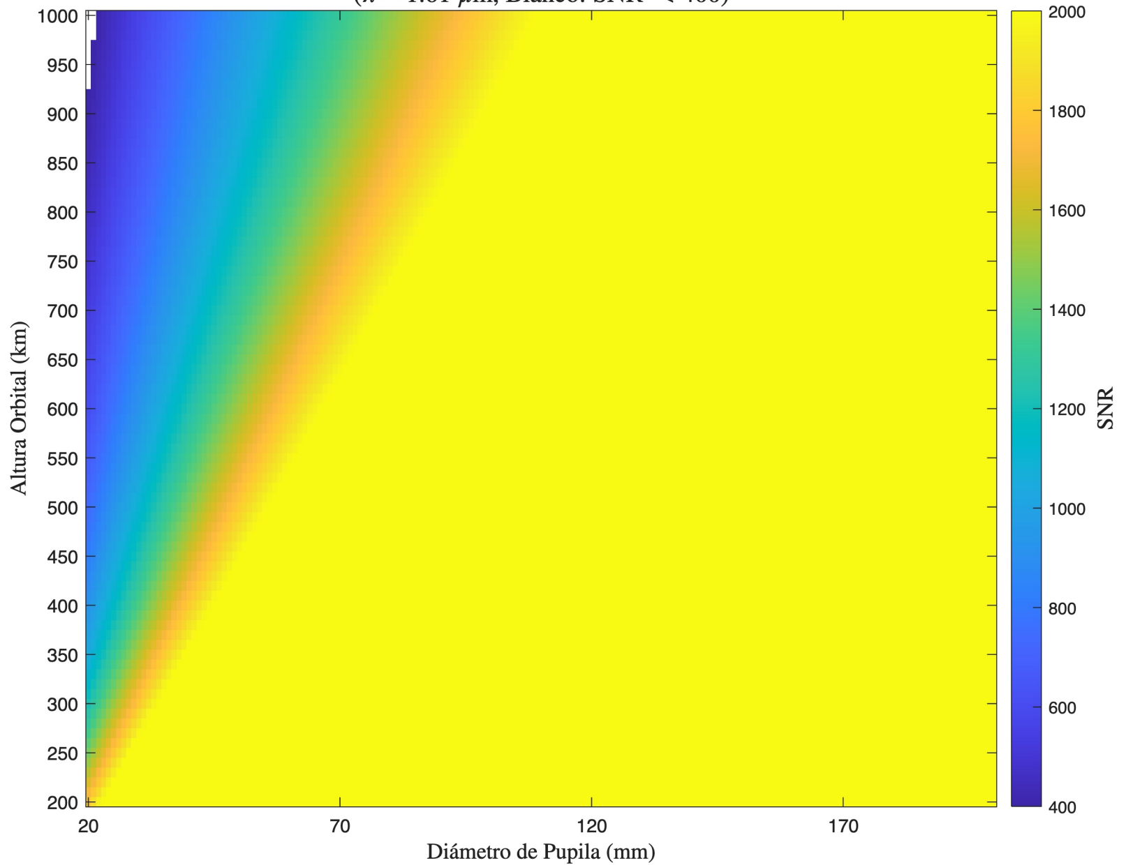
SNR - TMA - Detector 1 ( \lambda = 1.61 \mu\text{m} , Blanco: SNR < 400)
