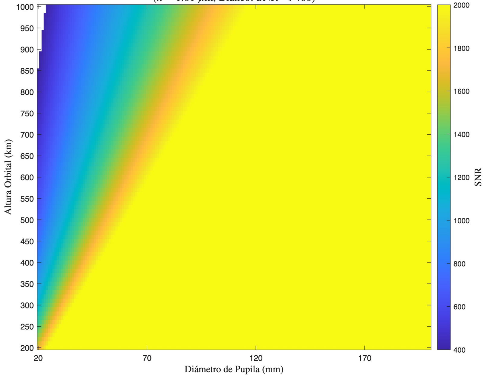
SNR - Korsch - Detector 2 ( \lambda = 1.61 \mu\text{m} , Blanco: SNR < 400)
